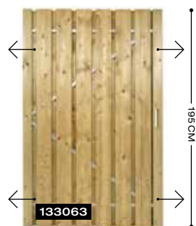
Vuren deur, stalen frame, universeel, 195 x 120 cm.
