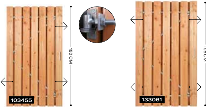
Douglas deur, stalen frame, geschaaft, universeel, 180 x 100 cm. Douglas deur, stalen frame, geschaaft, universeel, 195 x 120 cm.
