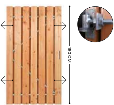
147302 geschaaft, universeel, 180 x 100 cm. 147305 ruw, universeel, 180 x 100 cm.
