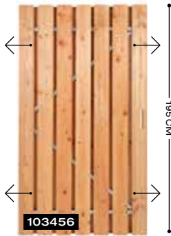
Douglas deur, stalen frame, geschaaft, universeel, 195 x 100 cm.
