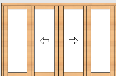
SD300 3000 x 1935 (schuif)
