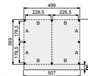
Douglasvision buitenverblijf basis 500x400 cm
