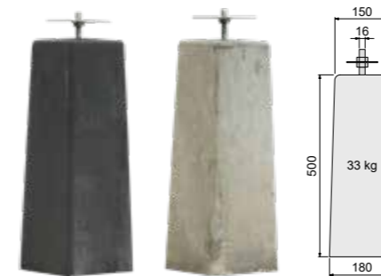
Betonpoer antraciet en grijs
