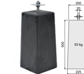
Betonpoer XL
