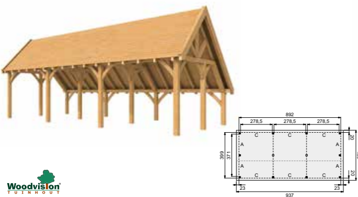
Douglasvision Kapschuur New Prestige 900x400 cm
