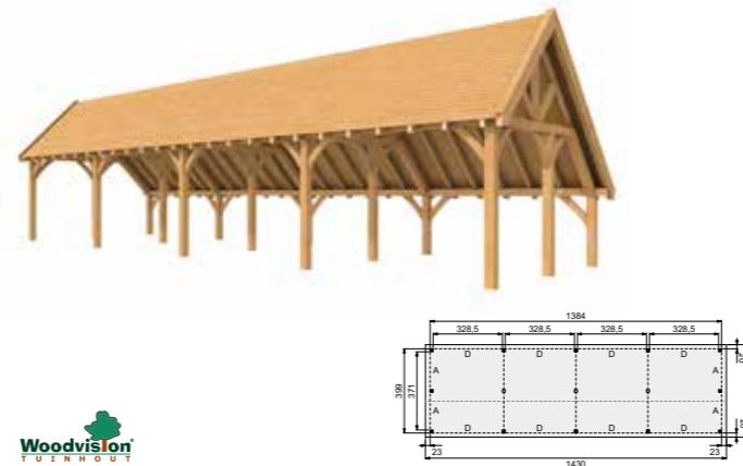
Douglasvision Kapschuur New Prestige 1400x400 cm
