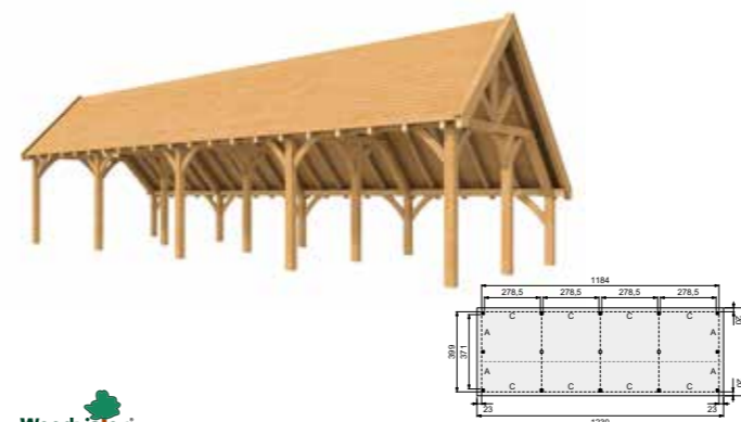
Douglasvision Kapschuur New Prestige 1200x400 cm
