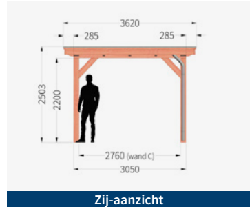
Zij-aanzicht
