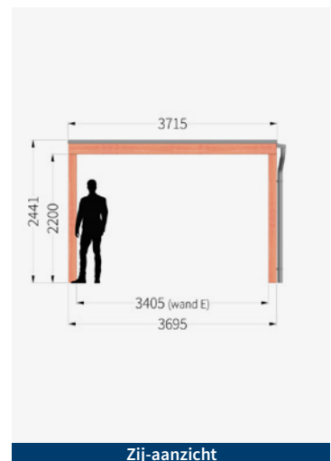
Zij-aanzicht
