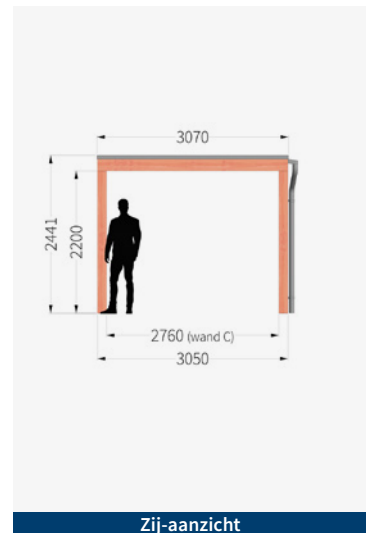
Zij-aanzicht
