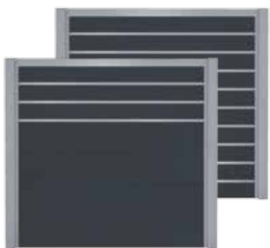
Alu RAL7016 10x WPC-vulling / RAL9006 met 3x Alu decorlijsten Art.9015 180 x 180 cm Alu RAL7016 10x WPC-vulling / RAL9006 met 9x Alu decorlijsten Art.9016 180 x 180 cm
